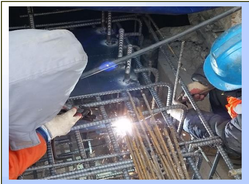
5STEP 앵카볼트 용접
